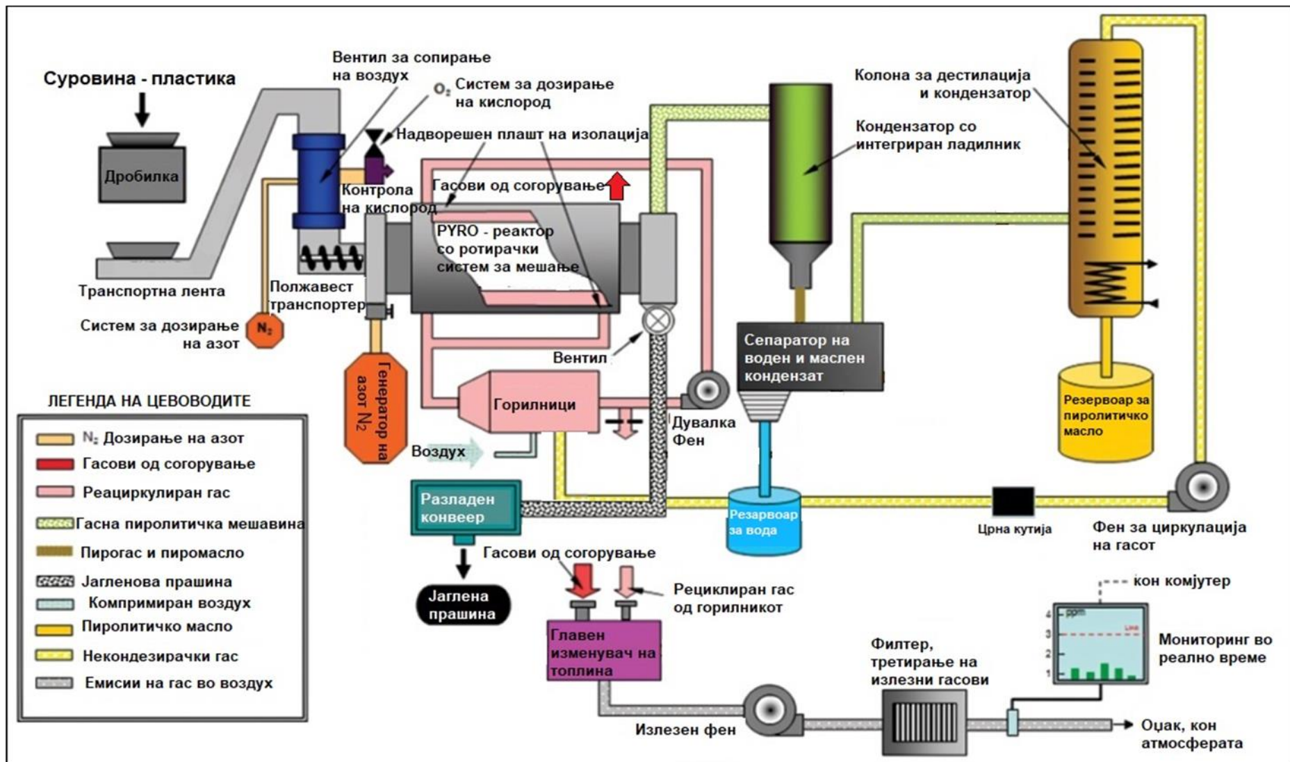
Слика 1. Поедноставен дијаграм на процесот на термичка декомпозиција на пластика
